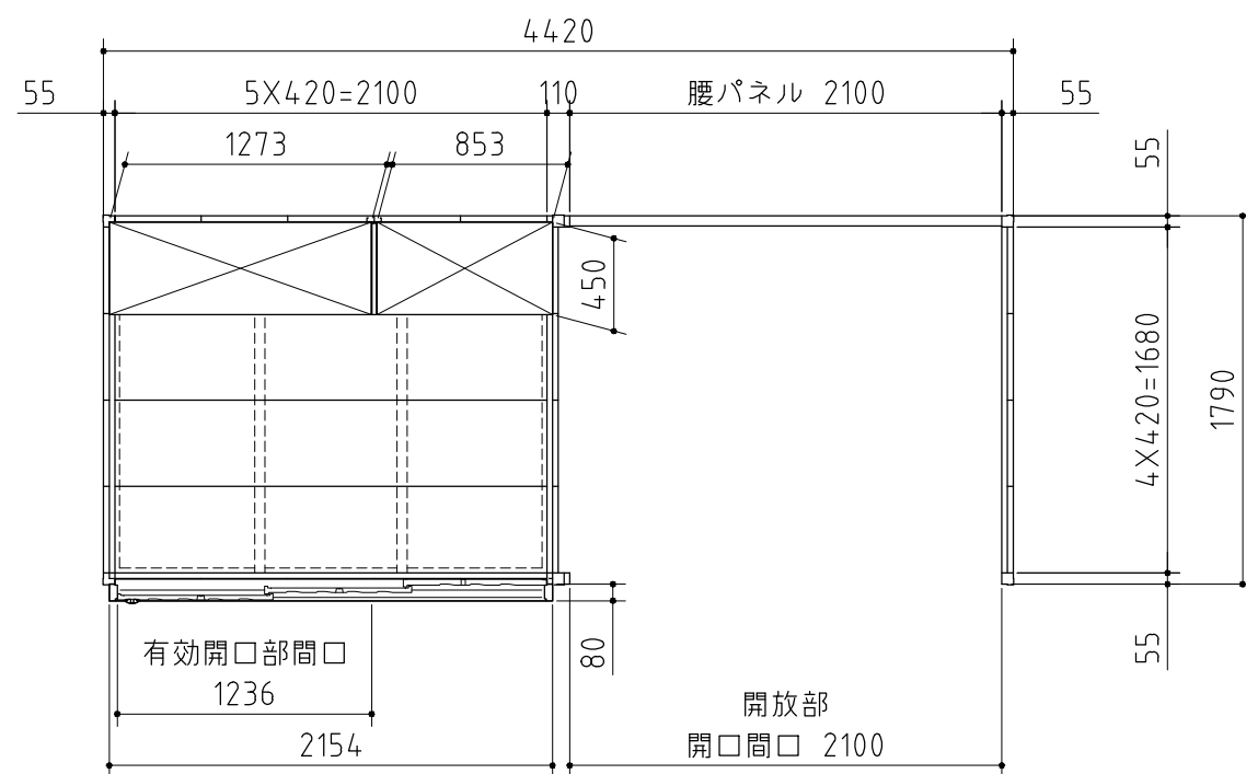
平面図
