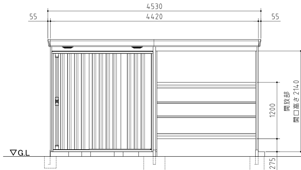
正面図
